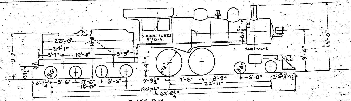
CLASS D-4 ENGS. NOS. 2201-2206
